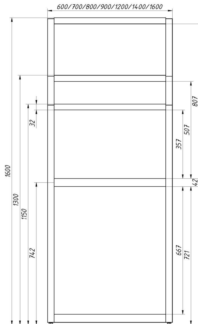
Размеры перегородок
