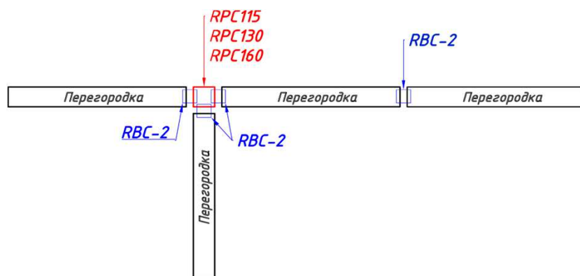
Крепление столешниц
